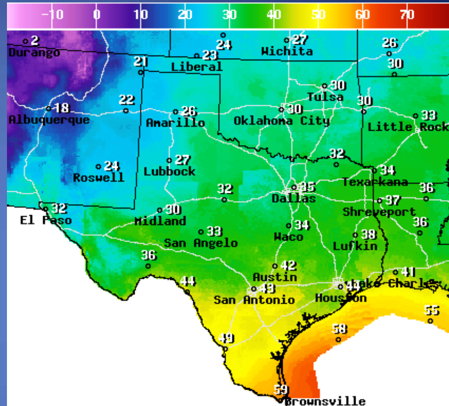
Temperature(F) For Sat Jan 28 2017 4AM EST (Sat Jan 28 2017 09Z)
