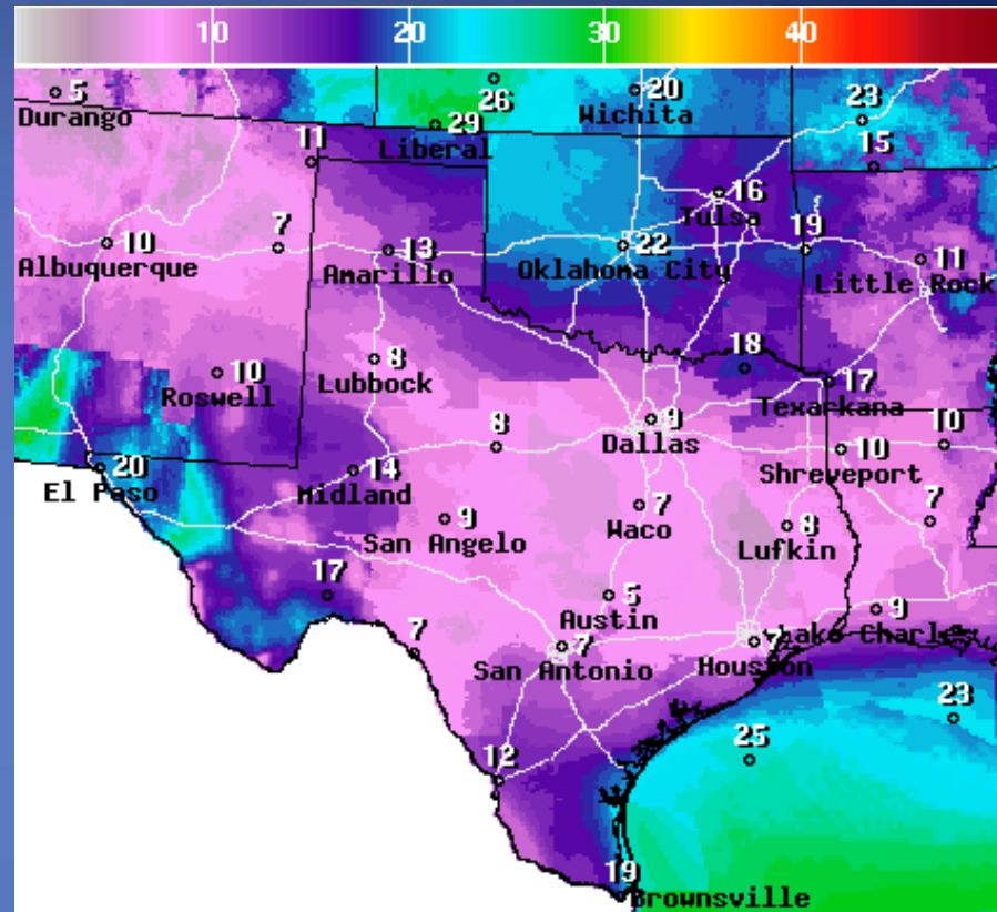
Wind Gust(Kts) Fri Jan 27 2017 4PM EST (Fri Jan 27 2017 21Z)
